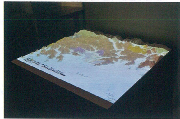
(赤穂コールドロン3D模型：海洋科学館)
