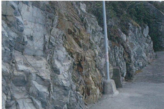
(噴火により噴出したマグマが固まった痕跡：御崎)
